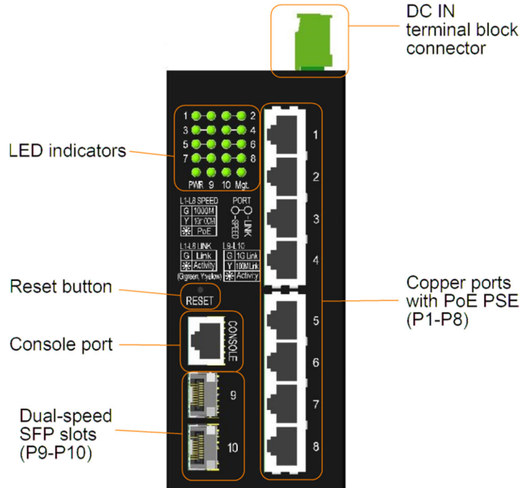
Frontblende
